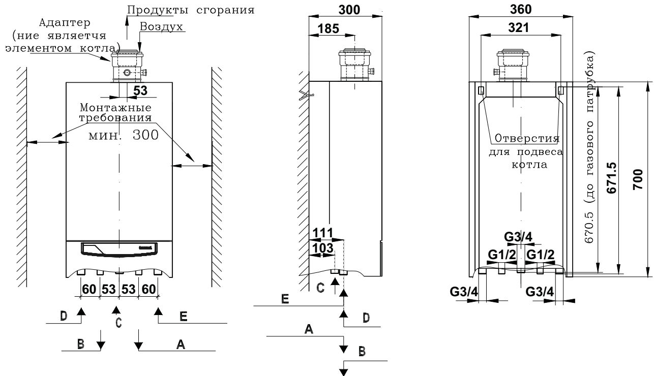
Рис. 3.3.1 Установочные размеры газового аппарата GCO-DP-21-23
