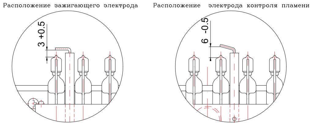
Рис. 6.1.2.1. Расположение электрод в горелке
