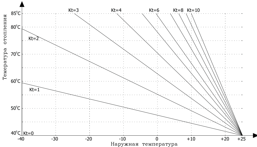
Рис. 2.4.1.1.1. Кривая нагрева
