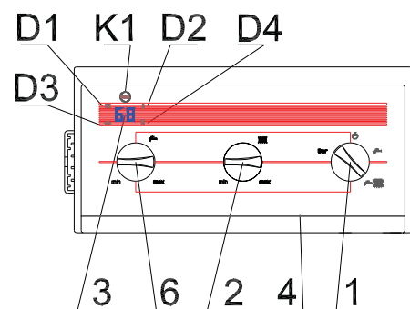
Рис. 5.2.1. Панель управления
